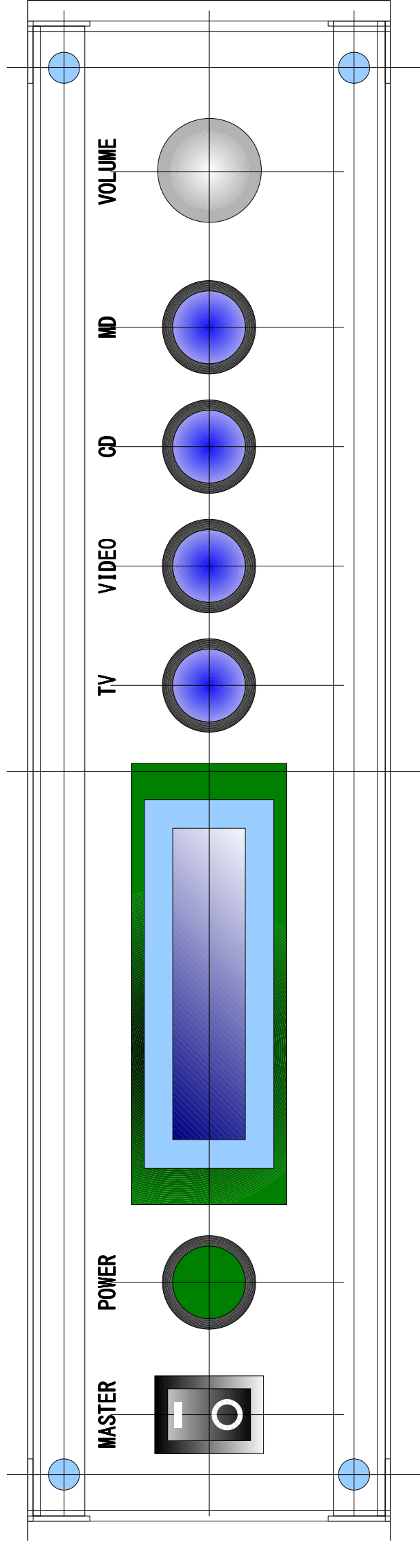
KLK-C1 フロントパネルレイアウト (原寸)
