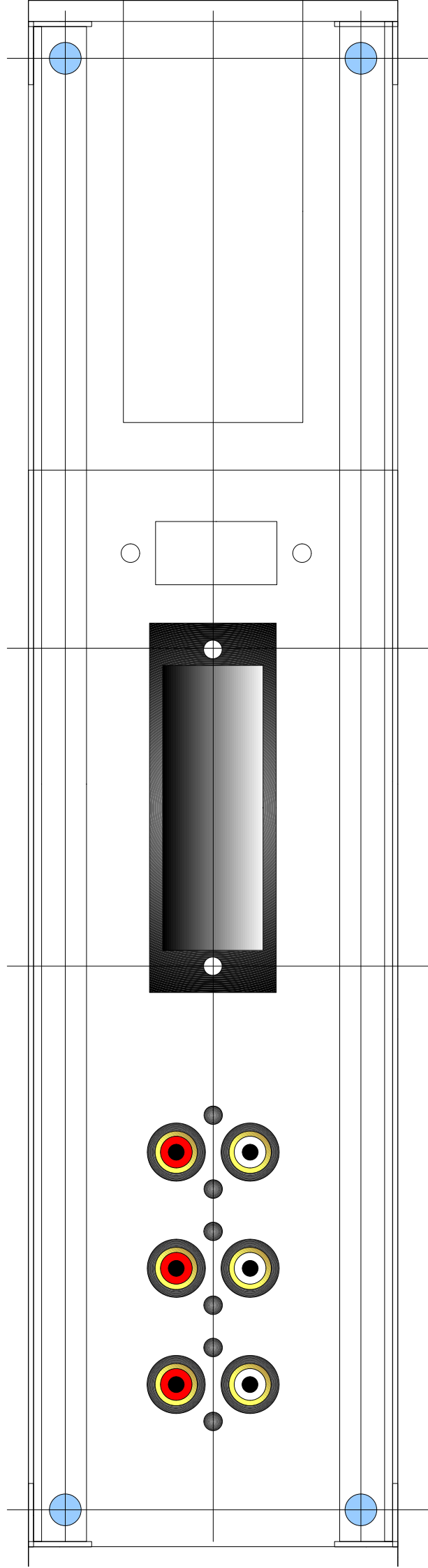
KLK-C1 リアパネルレイアウト (原寸)
