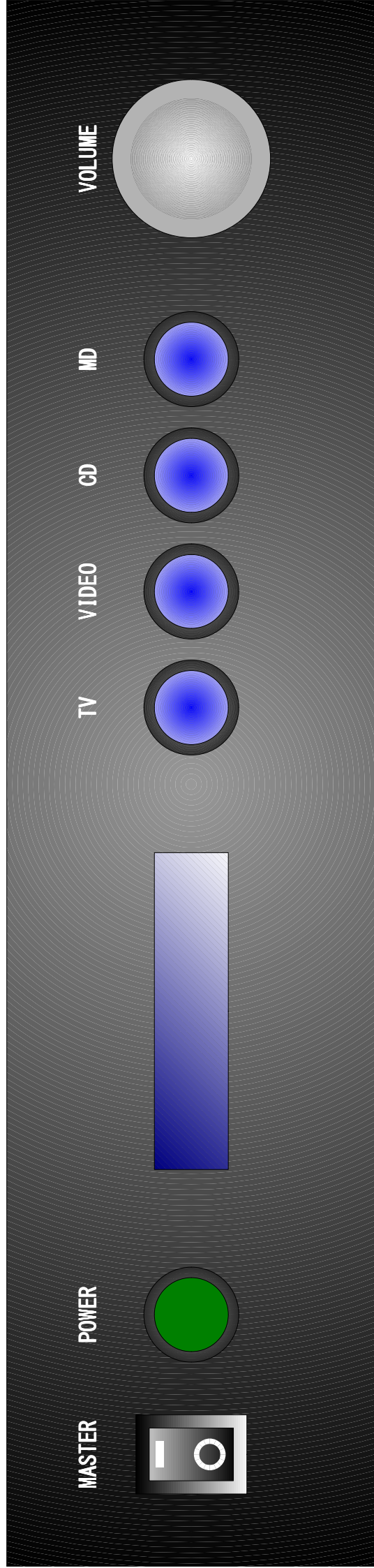
KLK-C1 フロントパネルシートデザイン (原寸)
